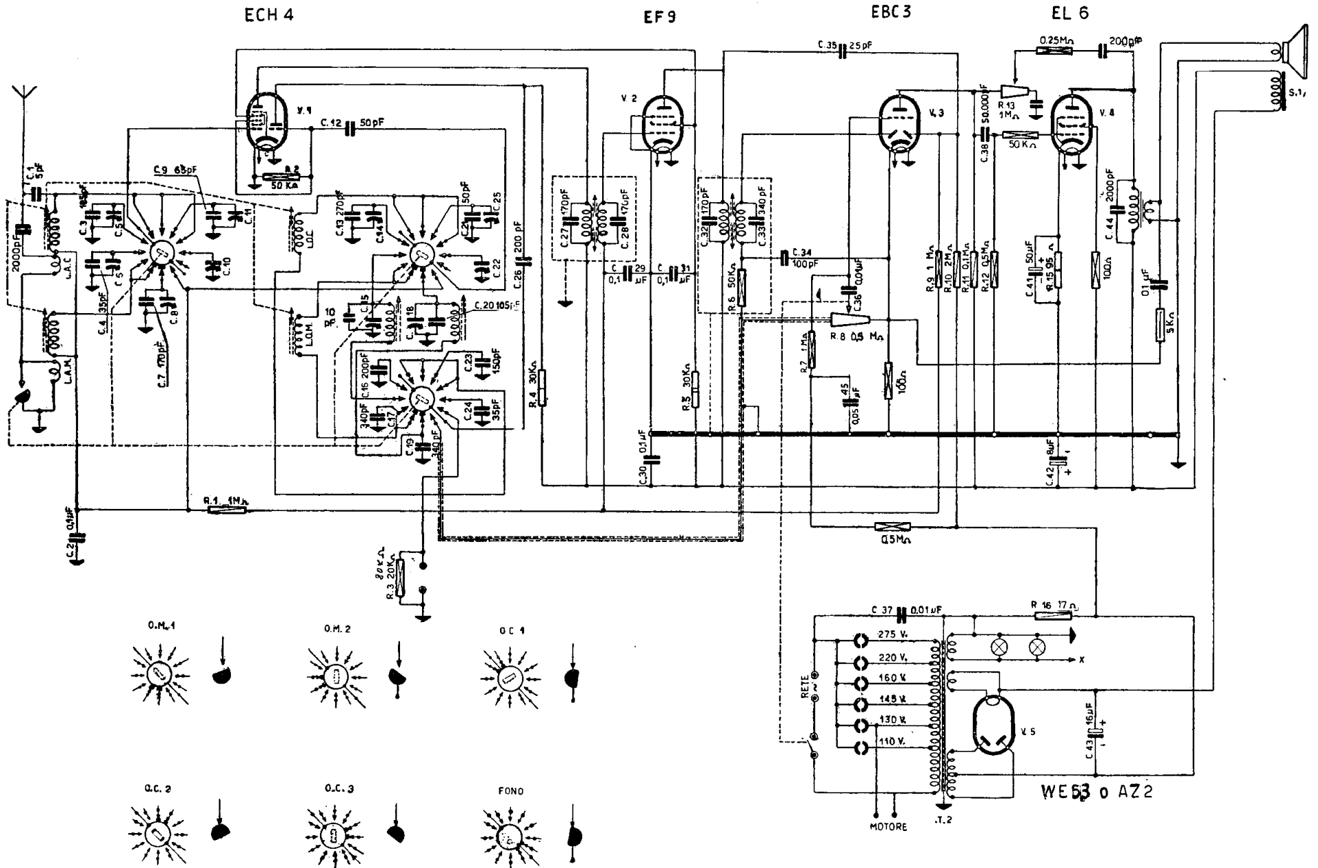
VOCE DEL PADRONE - Modd. 509, 519, 520 e 539 - Gamma onde medie divisa, e tre gamme onde corte divise e spostate. Media frequenza 465 kc. Il mod. 520 è con valvole Rimlock.
